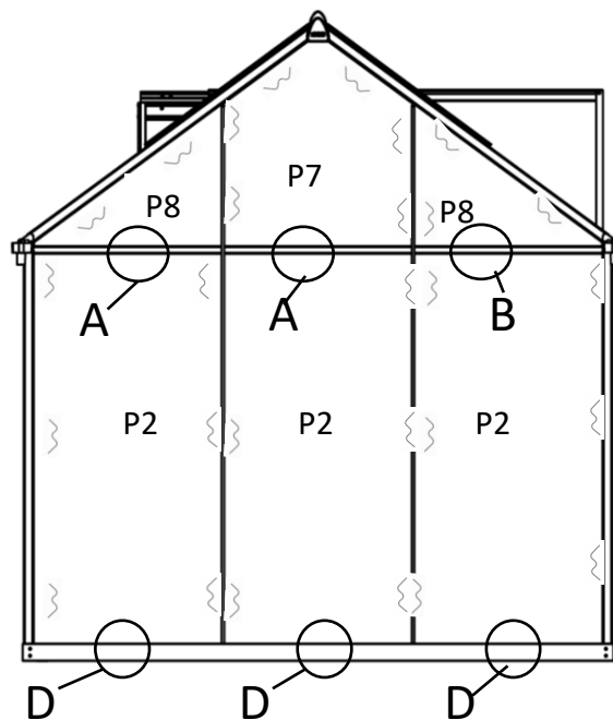
Rückansicht
