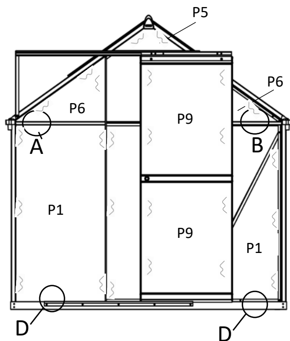
Vorderansicht
