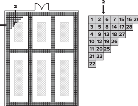
Abb. Nr. 6 Verlegung um feste Objekte herum – das Verfahren zum Verlegen von Fliesen
