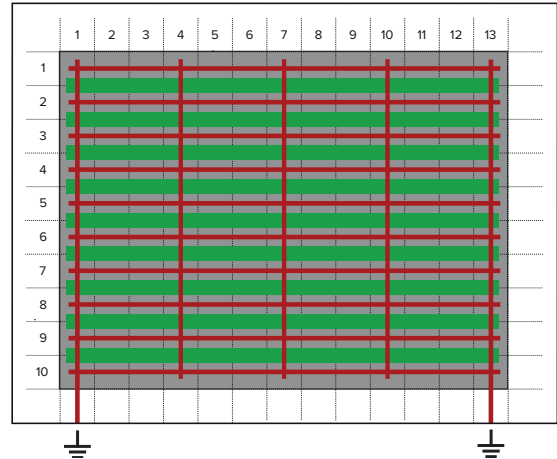
Abb. Nr. 4 Verlegung des Systems mit Fixierband.
