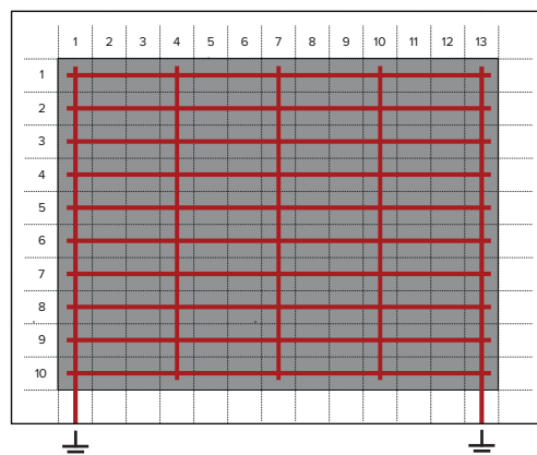
Abb. Nr. 5 Verlegung um feste Objekte – Linienmarkierung
