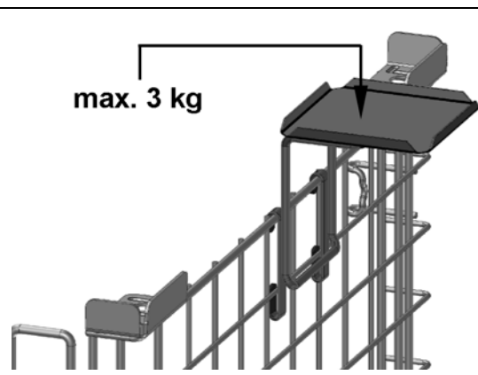
Bild 51 Alternativ-Montage
