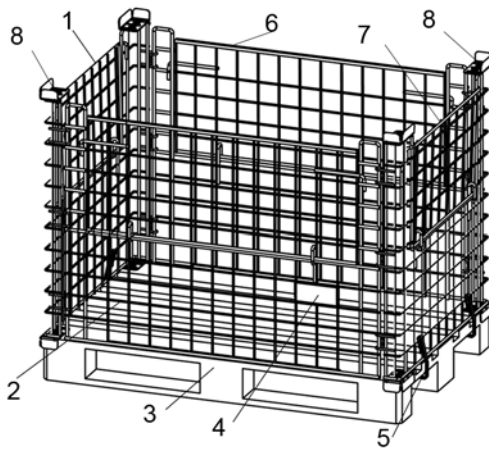
Bild 1 Palettenaufsatz stapelbar 1 = Seitenteil 2 = Vorderteil klappbar 3 = Euro- / Düsseldorfer Palette 4 = Typenschild 5 = Haltebügel 6 = Rückenteil klappbar 7 = Seitenteil klappbar 8 = Stapelecke
