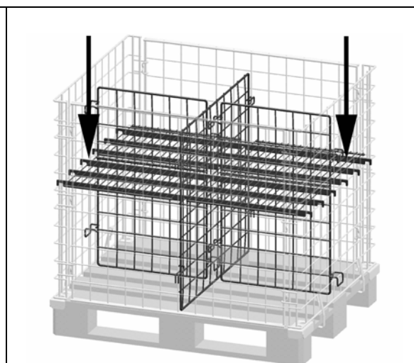
Bild 34 Böden einhängen.
