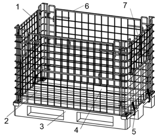
Bild 2 Palettenaufsatz nicht stapelbar 1 = Seitenteil 2 = Vorderteil klappbar 3 = Euro- / Düsseldorfer Palette 4 = Typenschild 5 = Haltebügel 6 = Rückenteil klappbar 7 = Seitenteil klappbar
