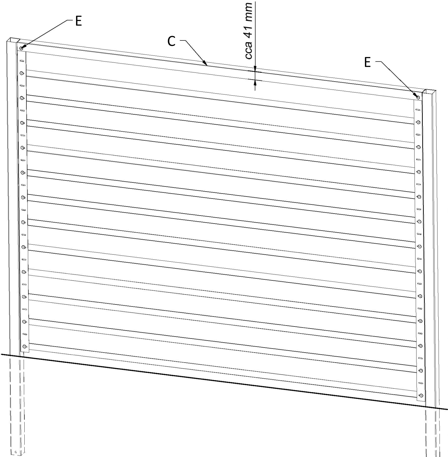
BLICK VON DER STRASSE street view
